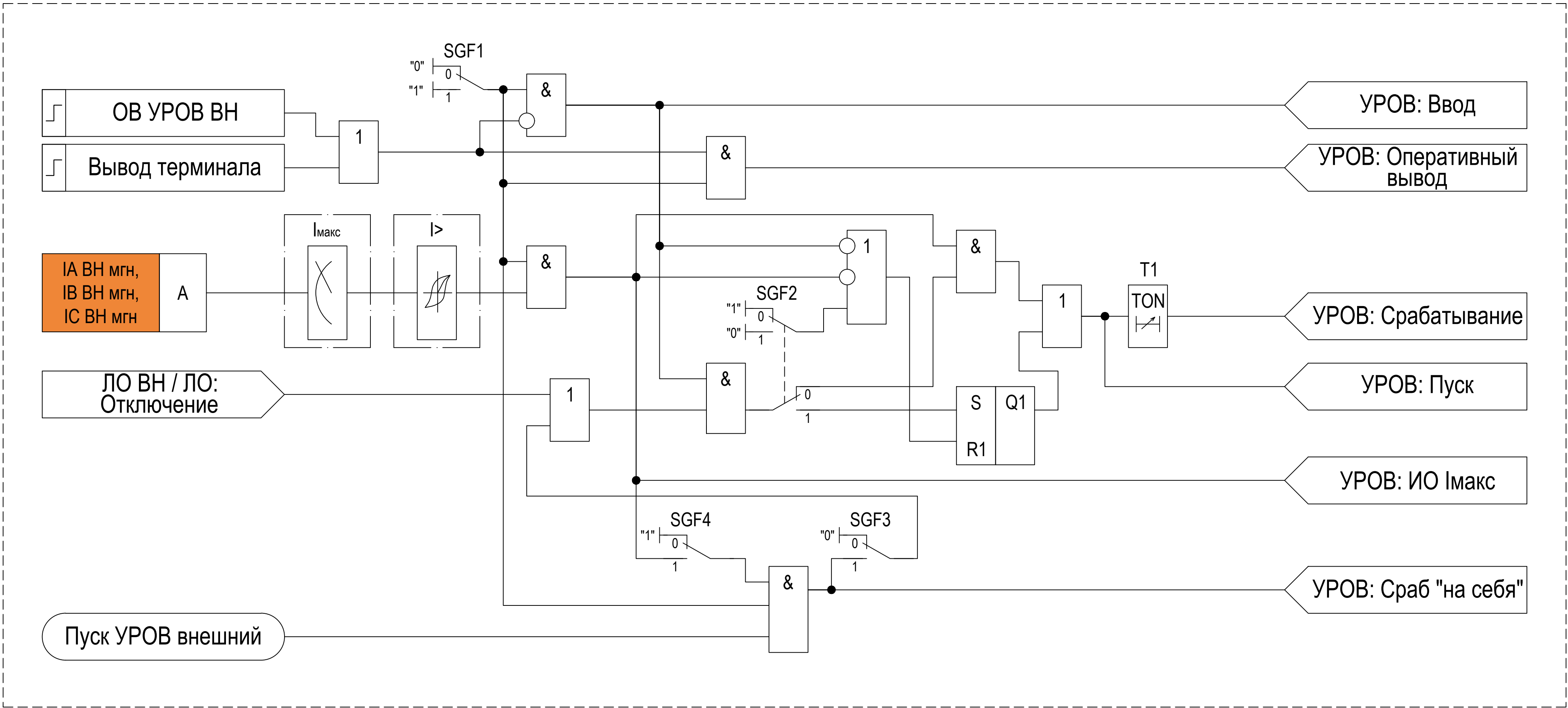
Устройство резервирования при отказе выключателя (УРОВ) (TPBRF) RBRF1
